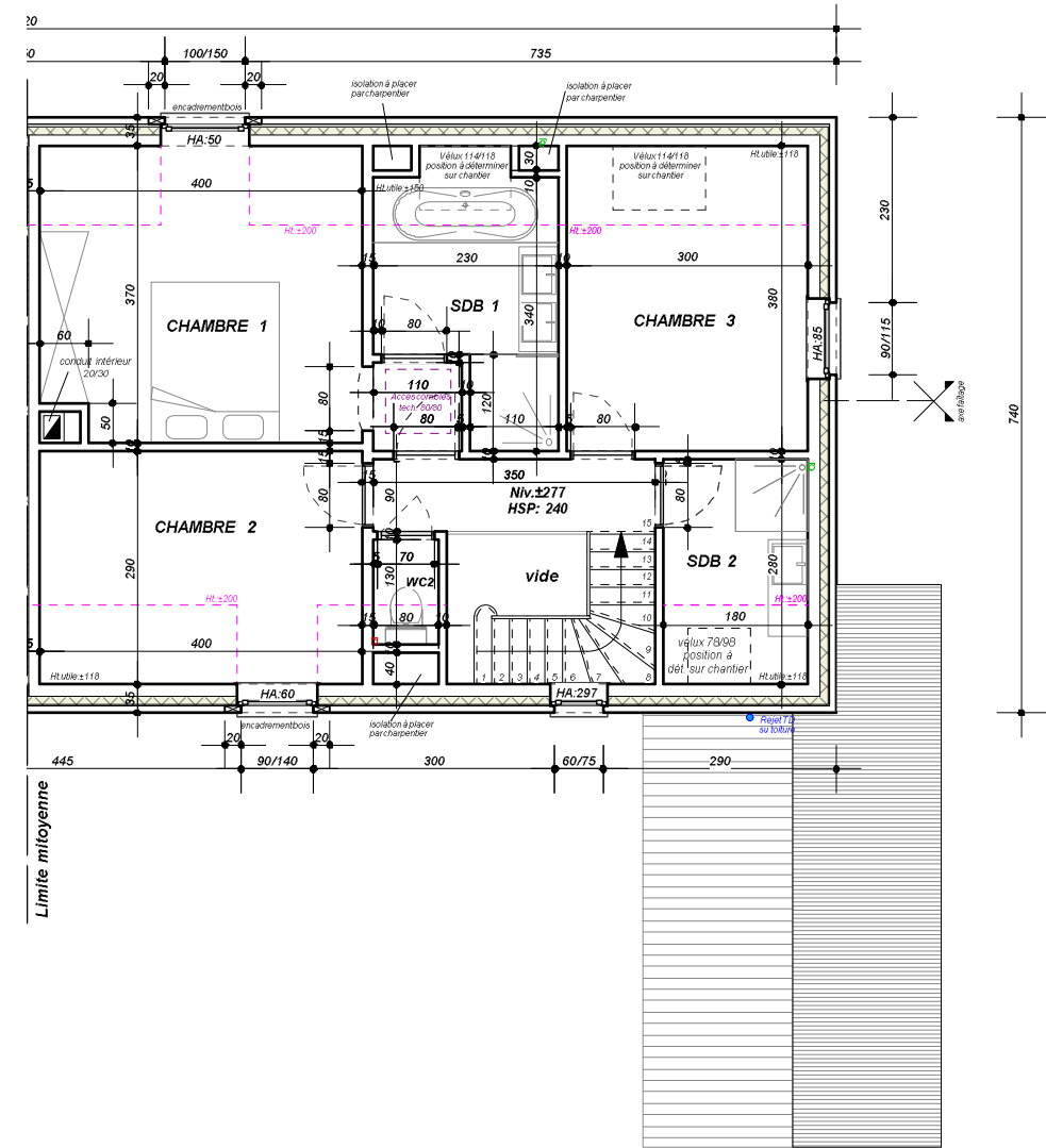
VUE EN PLAN ÉTAGE
