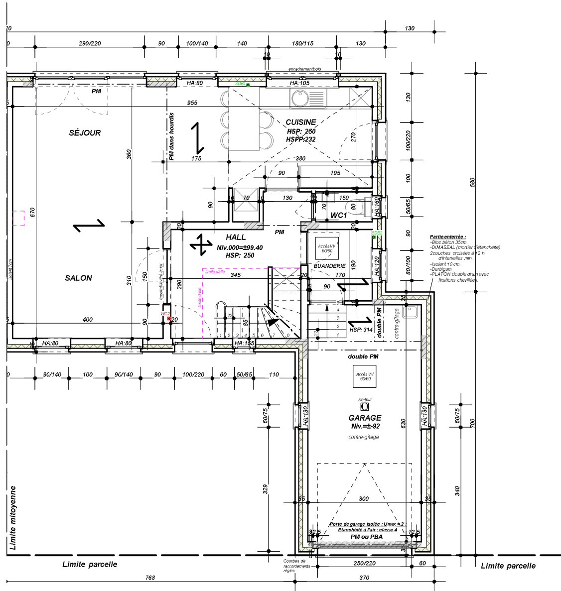
VUE EN PLAN REZ DE CHAUSSEE
