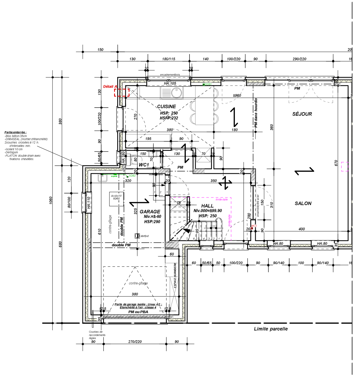
VUE EN PLAN REZ DE CHAUSSEE
