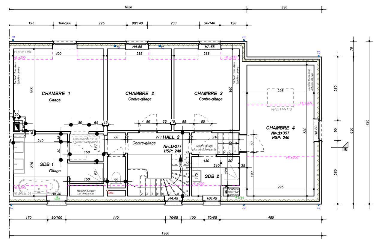
VUE EN PLAN ÉTAGE
