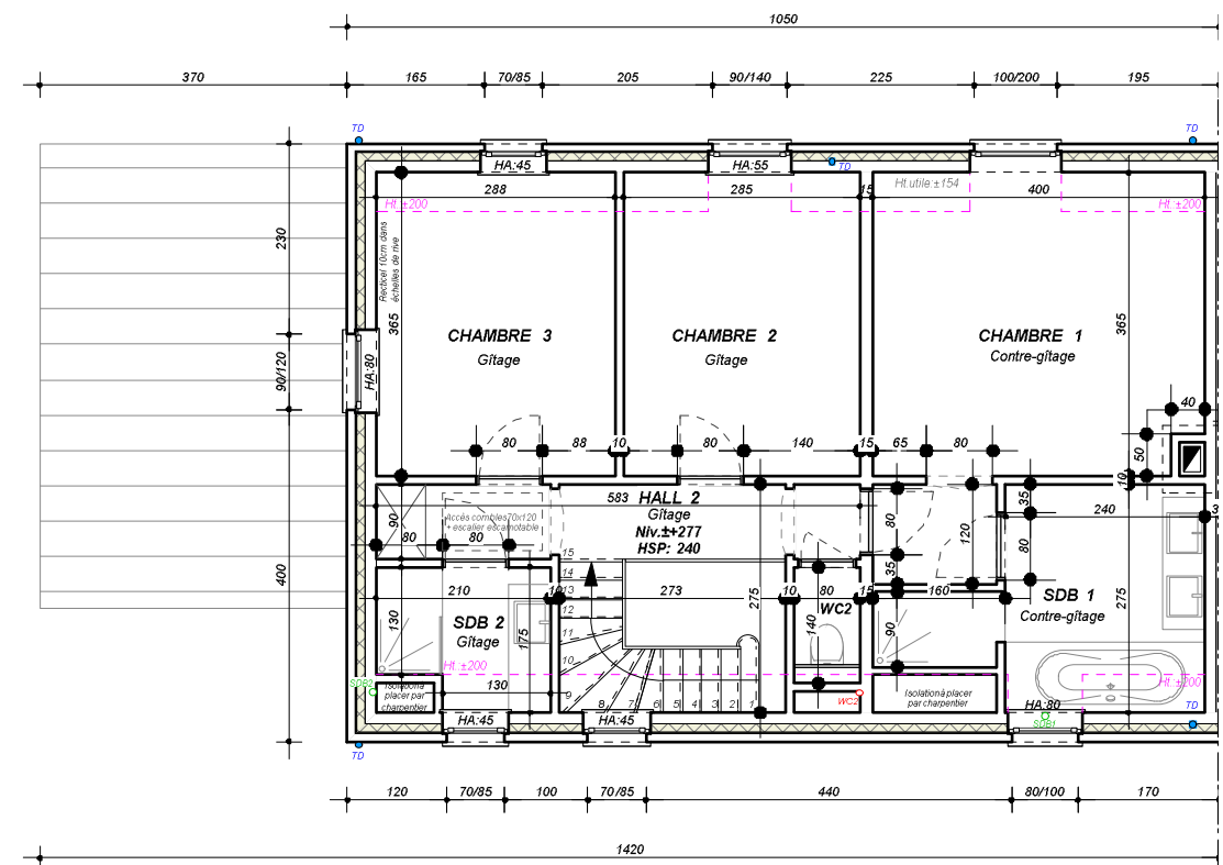
VUE EN PLAN ÉTAGE
