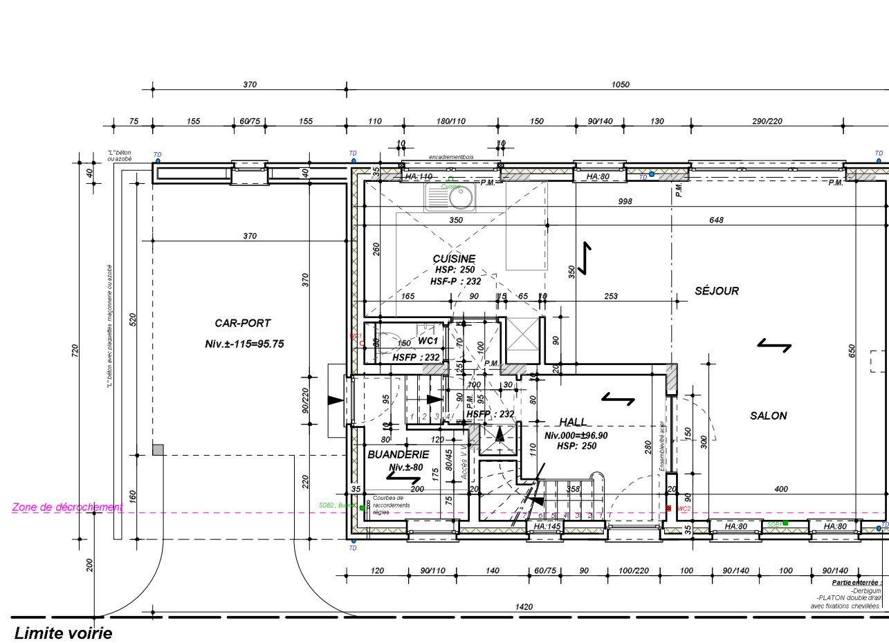
VUE EN PLAN REZ DE CHAUSSEE
