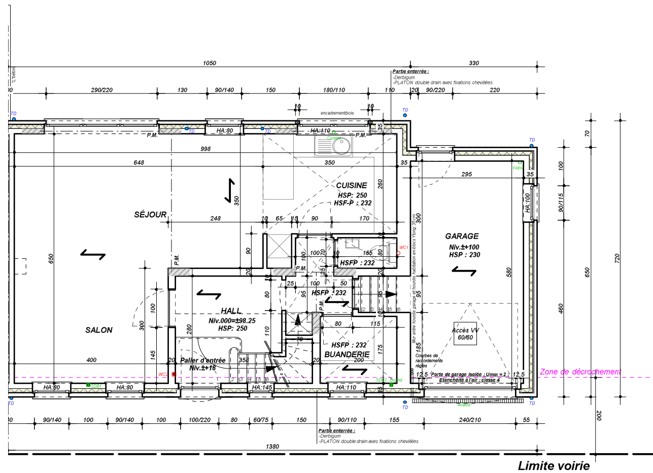
VUE EN PLAN REZ DE CHAUSSEE
